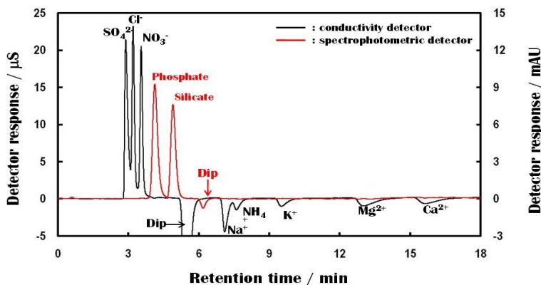
図1 弱酸性陽イオン交換型カラムと導電率型検出器、ポストカラム誘導体化法-吸光検出器を組み合わせた主要陰イオンおよび陽イオン、リン酸、ケイ酸の同時分離測定法による河川水試料の測定例。
