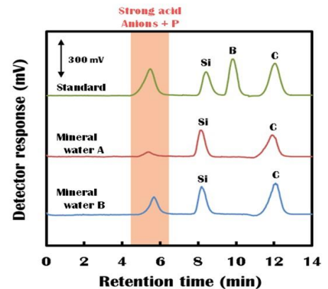
図2 イオン排除型イオンクロマトグラフ/荷電化粒子検出器によるケイ酸、ホウ酸、炭酸の同時分離測定例。
